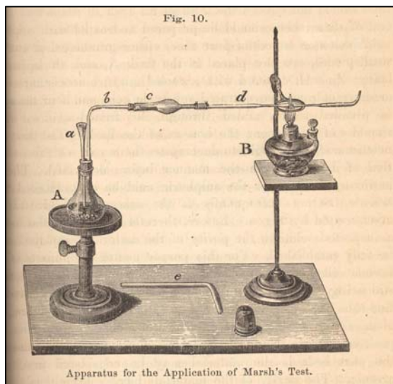
Figura 1 - Aparelho de Marsh
